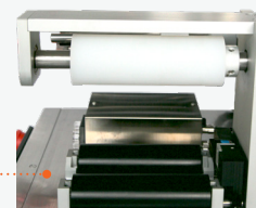
自動感應啟動電眼 & 快速調整扶瓶滾輪座 Labeling start-up sensor & Quick-changeover bottle holder
