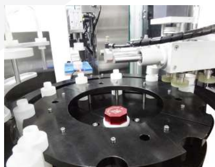
星盤機構 Indexing system
